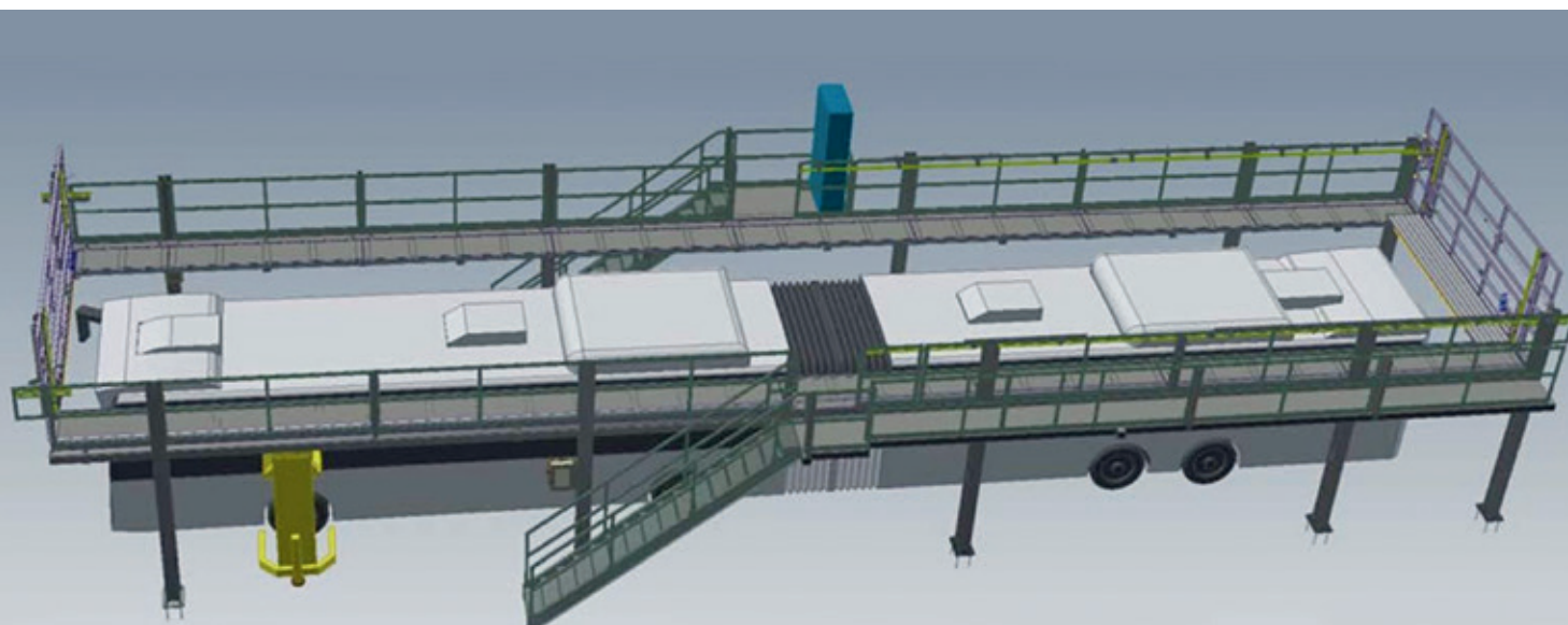
Prinzipskizze der Arbeitsbühnen des Dacharbeitsstandes (Ebene +1)
